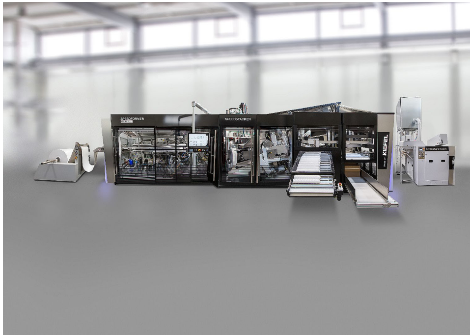
Die becherformende Maschine KTR 5.2 SPEED bietet Produktionssteigerung und maximale Effizienz. © KIEFEL GmbH
